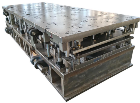
順送板金プレス金型
