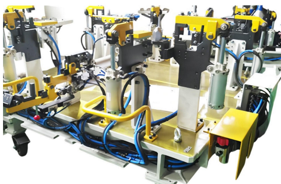
固定具
